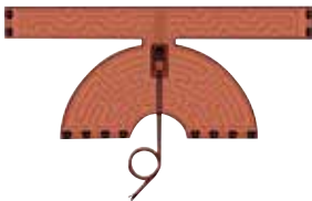
Fascia riscaldante per tramoggia 8.5 L Heating belt for 8.5 L hopper 12.X5
